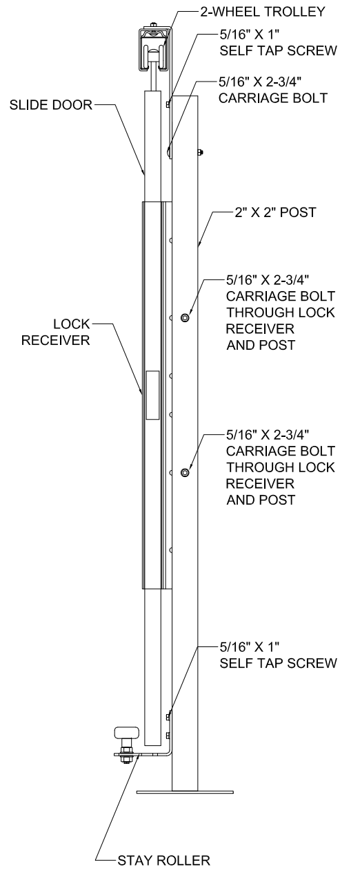
SLIDE DOOR SIDE
